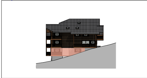
Façade EST
